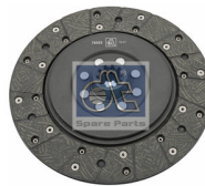
Koppelingsplaat, 250 mm repl. Sachs: 1861 291 136 DT 4.64262 · repl. Mercedes 014 250 9403
